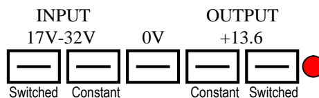
PV3s-A Connections
