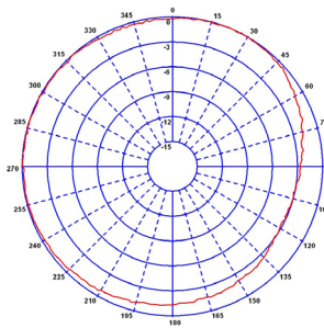
H-Plane (390MHz)
