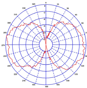
E-Plane (390MHz)
