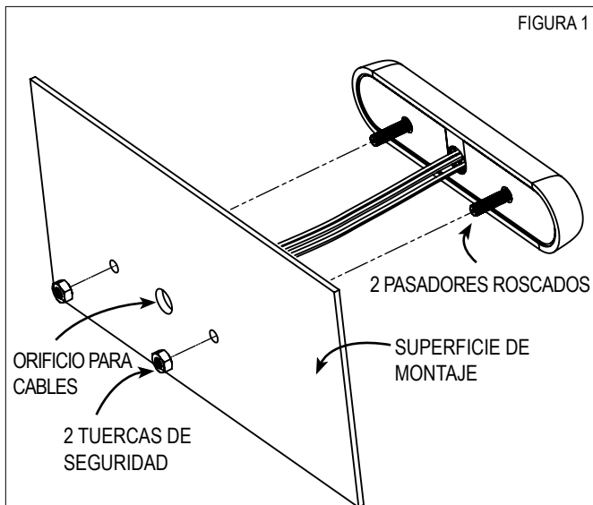
MONTAJE CON PASADORES - ROSCADOS (MOSTRADO) FORD GRILLE MONTAJE- ROSCADOS (SIMILAR, NO SE MUESTRA)
